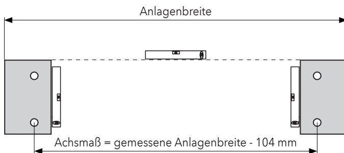
Konsolenanordnung Wandmontage
