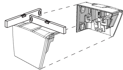
Waagerechte Konsolenausrichtung
