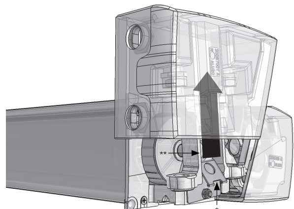
Abb. 10: Federmechanismus* und Führungskanal** beim Einhängen beachten
