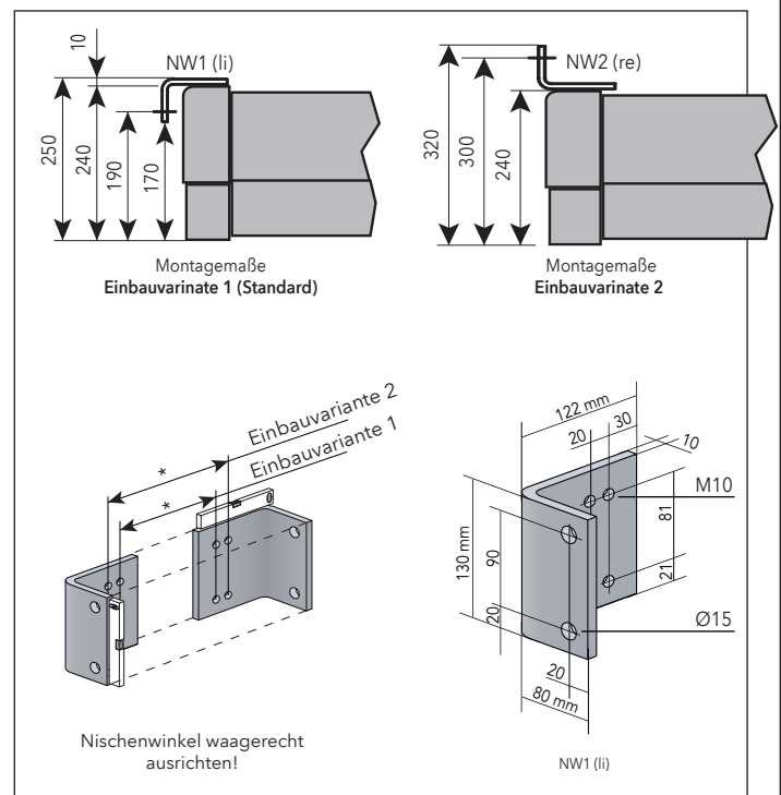
Abb. 17: Nischenwinkel und Montagemaße
