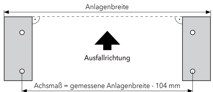
Konsolenanordnung Deckenmontage
