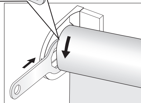
Obere Endlage nach oben verstellen Réglage du fin de course haut vers le haut Adjust top end position upwards
